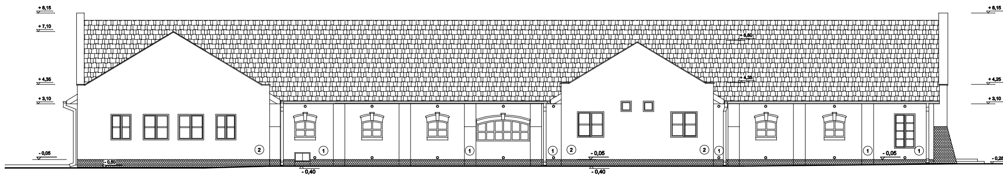
ELEWACJA PÓŁNOCNA
