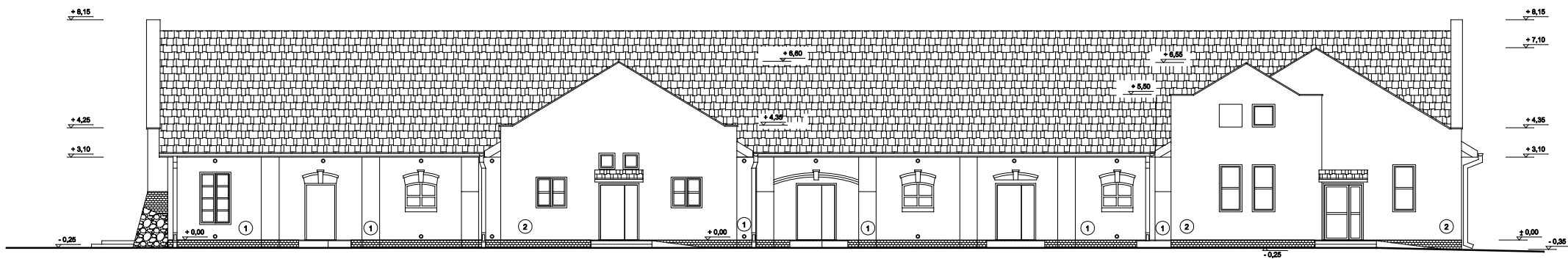
ELEWACJA POŁUDNIOWA
